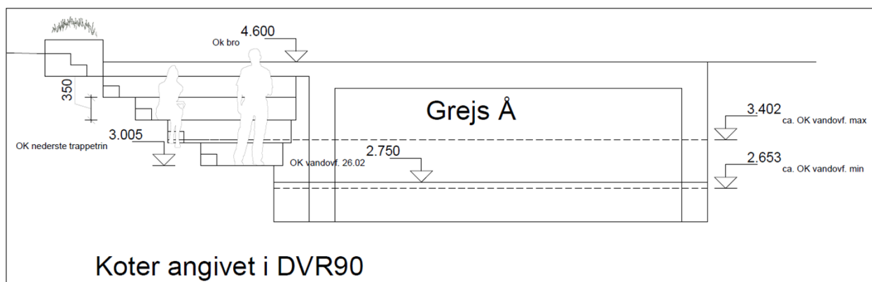
Figur 2 - Tværsnitstegning
